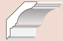
BMCR 806 8 1/4" W x 5 1/16" H x 5 1/4" D
